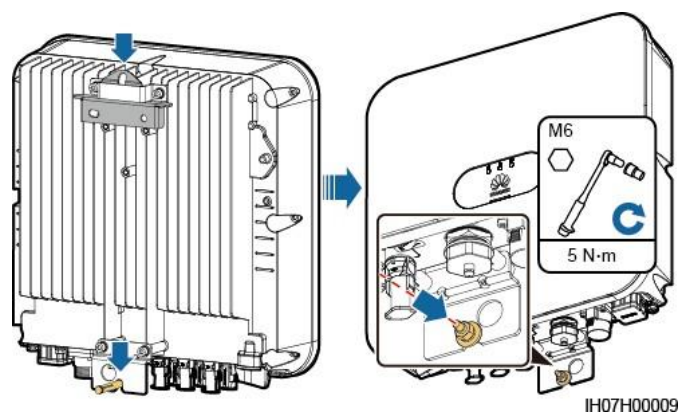
4-11. ábra Az anyák meghúzása
