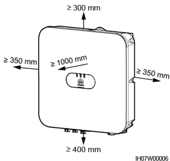
4-2. ábra Telepítési térszükséglet
