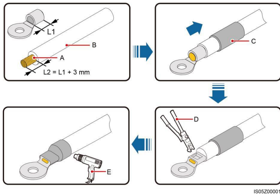
5-2- ábra OT kivezetés krimpelése
