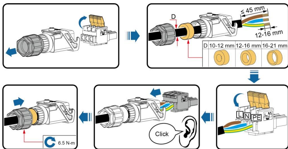
5-7. ábra AC csatlakozó összeszerelése (háromeres vezeték)
