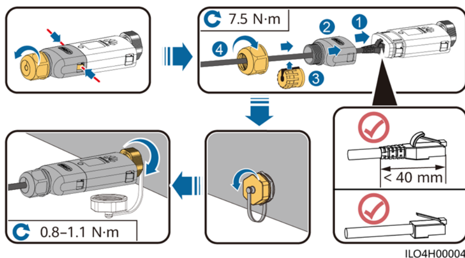
5-15 ábra WLAN-FE Smart Dongle beszerelése (FE kommunikáció)
