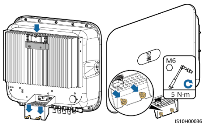
4-11 ábra A SUN2000 telepítése
