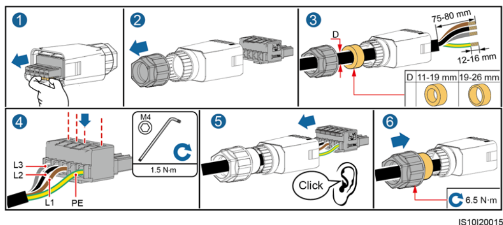
5-7 ábra Négyeres kábel (L1, L2, L3 és PE)
