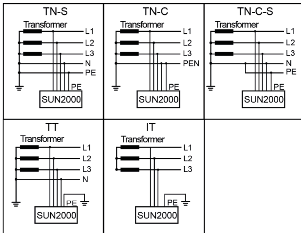
2-4 ábra Támogatott villamos hálózatok
