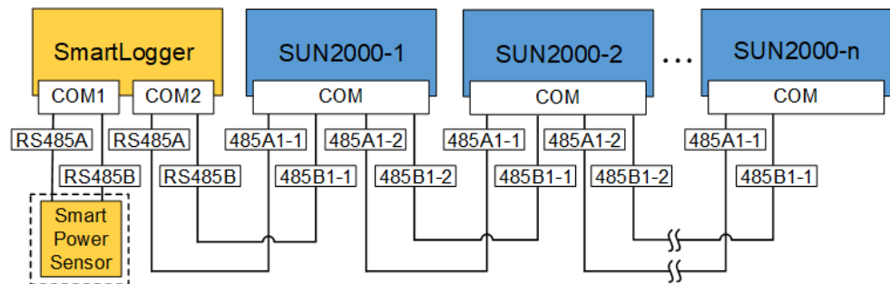
5-19 ábra SmartLogger naplózó hálózati leosztás
