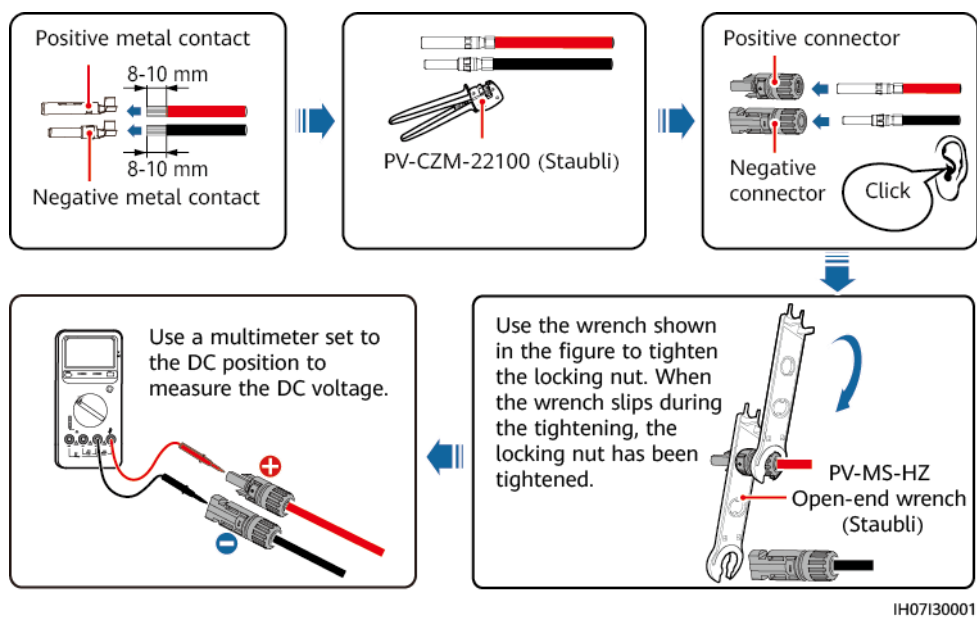
5-13 ábra A DC csatlakozó összeszerelése
