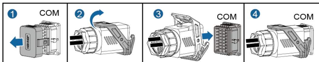
5-21 ábra A jelkábel csatlakozójának rögzítése
