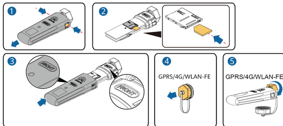
5-16 ábra A 4G Smart Dongle beszerelése
