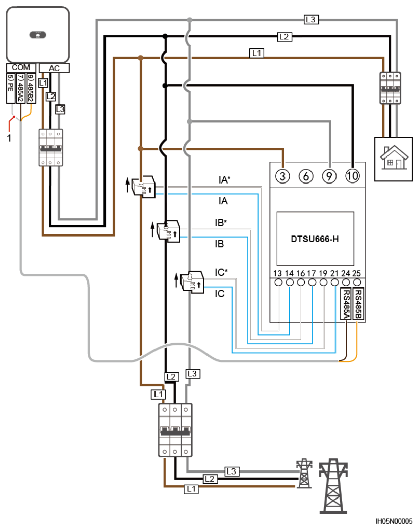
5-22 ábra Kábelcsatlakozás (háromfázisú, háromkábeles)
