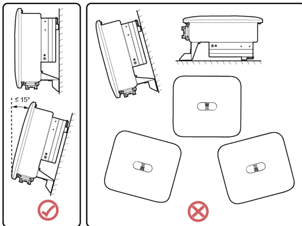
4-1 ábra Beszerelési dőlés
