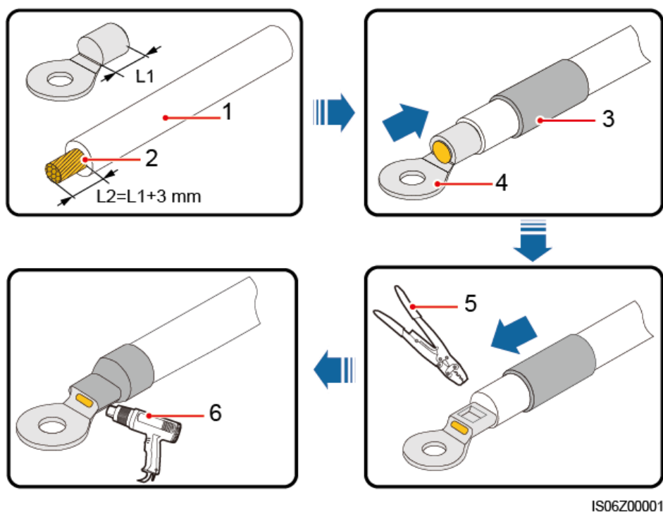
5-2 ábra OT saru krimpelése
