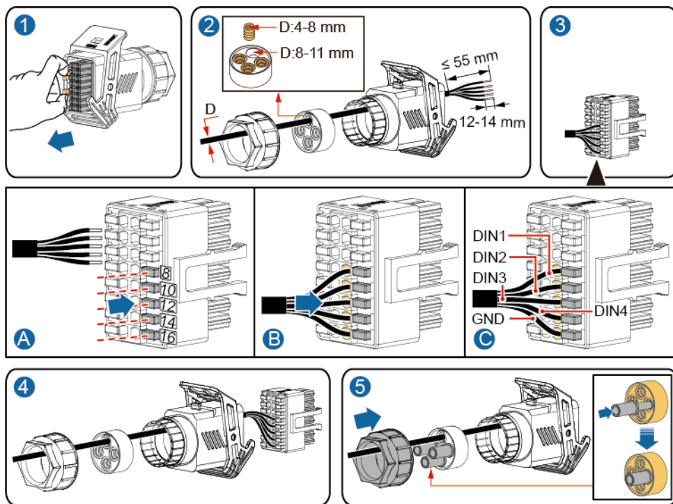
5-29 ábra A jelkabel telepítése
