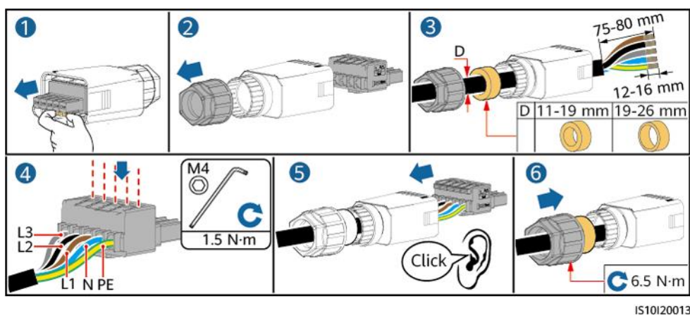
5-9 ábra Ötteres kábel (L1, L2, L3, N és PE)
