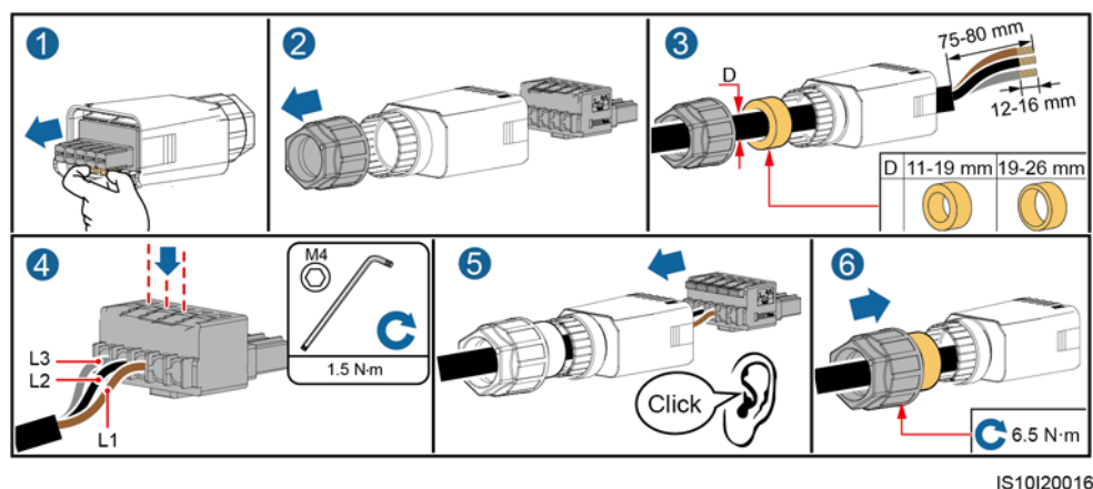
5-6 ábra Háromeres kábel (L1, L2 és L3)
