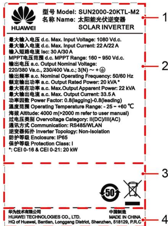
2-6 ábra Adattábla (SUN2000-20KTL-M2 példaként használatos)
