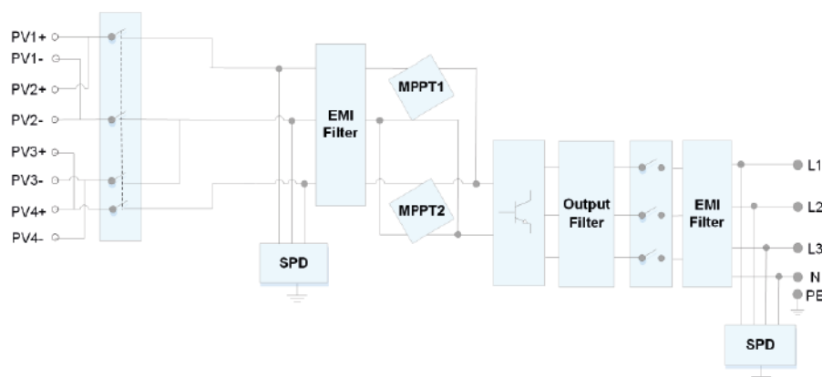
2-7 ábra A SUN2000 koncepció ábrája
