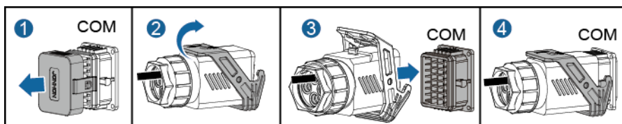
5-30 ábra A jelkabel csatlakozójának rögzítése
