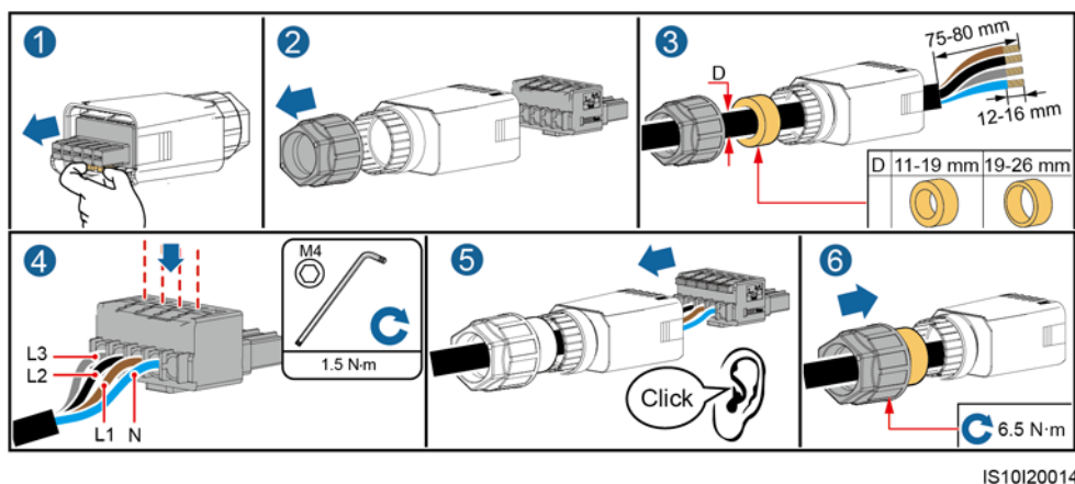
5-8 ábra Négyeres kábel (L1, L2, L3 és N)
