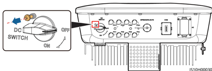
6-1 ábra A DC kapcsolót rögzítő csavar eltávolítása
